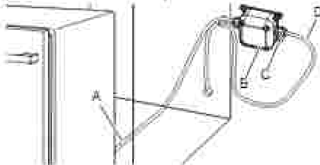
A. Câble du boîtier de raccordement électrique B. Boîtier de raccordement électrique C. Raccord de câbles (2) D. Câblage domestique
